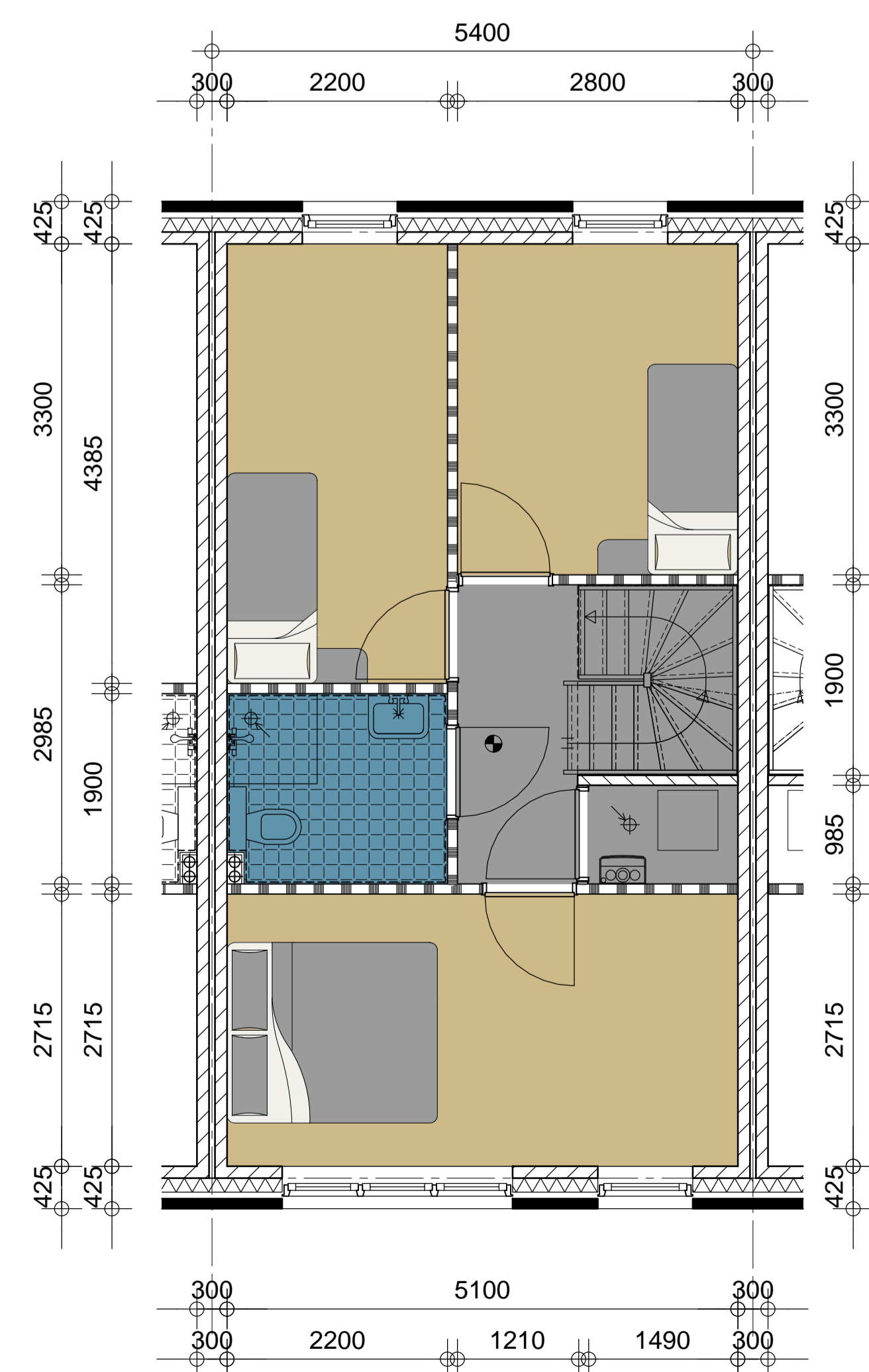
Verdieping
