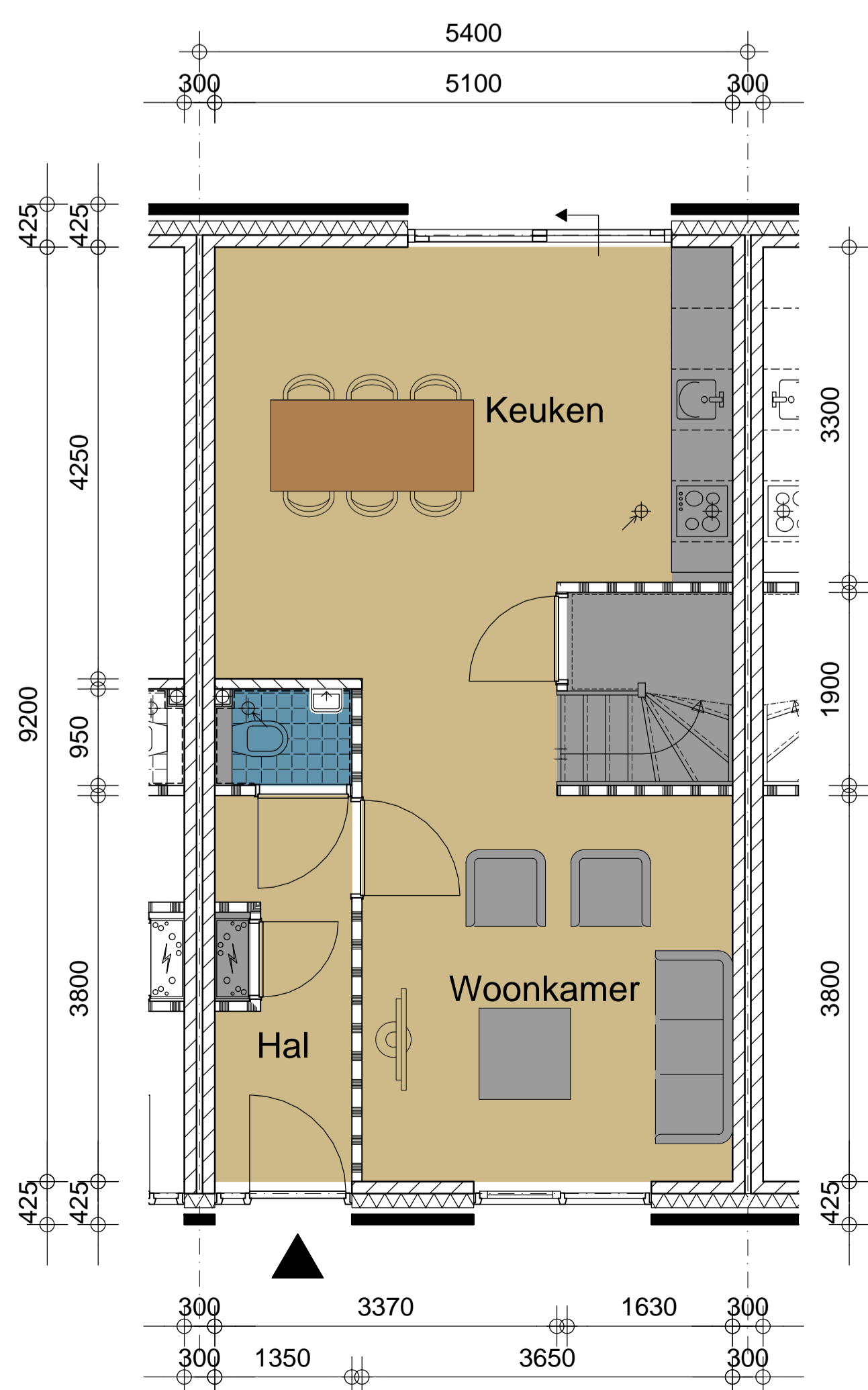
Begane grond
